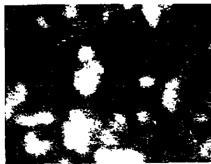
图 3 化学镀法加镍,镍在复合粉末中的分布状态(扫描电镜面扫描) \times 600
